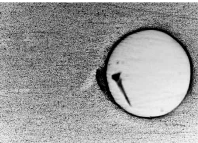
Rys. 7. Fotografia zglądu makroskopowego połączenia drut kanthal/aluminium. Widoczne połączenie na całym obwodzie wzmocnienia. Drut nie uległ deformacji. Pow. 200× [8]
